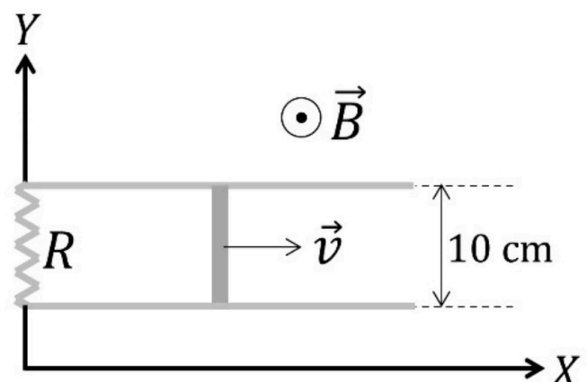
Figura 4.1. Varilla móvil.
